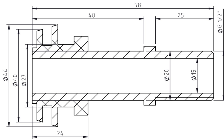
ŘEZ B-B MĚŘÍTKO 1:1
